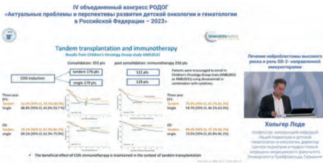
Рис. 5. Слайд № 5
