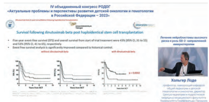
Рис. 6. Слайд № 6
